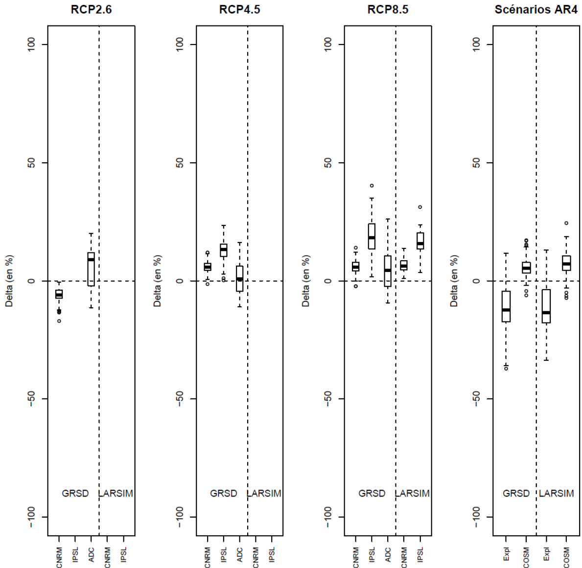
Figure 53 : Distributions des évolutions des débits simulés par les modèles GRSD et LARSIM pour le futur proche en utilisant trois projections climatiques AR5 (CNRM, IPSL et ADC) forcées par trois scénarios RCP (2.6, 4.5 et 8.5), et deux projections climatiques AR4 (issues d'Explore 2070 et COSMO-CLM), sur l'ensemble des bassins de la zone d'étude. 6 MCG sont inclus pour Explore 2070, et 3 réalisations pour COSMO-CLM. Les évolutions en pourcentage de l'ensemble des stations sont agrégées dans les boîtes à moustaches. A noter que ceci est une reprise de la Figure 29 (gauche) complétée avec les scénarios AR4.
