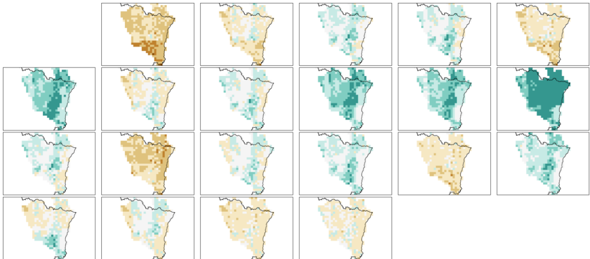
Figure 57 : Evolution de la précipitation annuelle moyenne en mm/j pour 21 modèles entre 2021-2050 et la période historique, données issues de l'ADC pour le RCP2.6.
