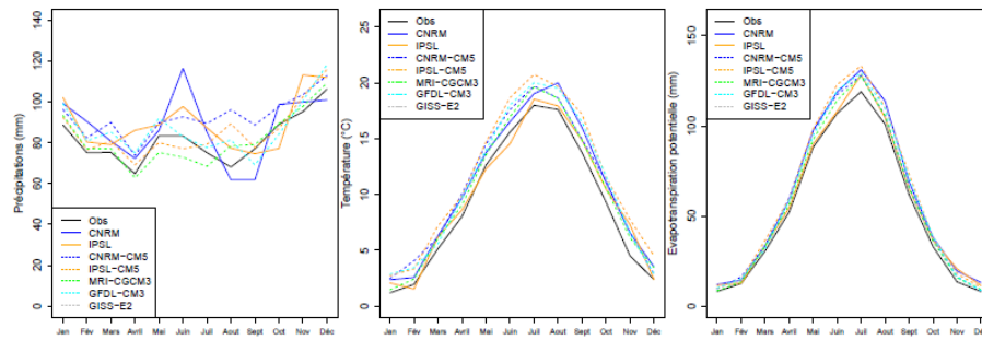
Figure 43 : Exemple de fiche climat pour la Moselle à Perl : extrait des indicateurs fournis pour une période future. Cas du RCP8.5 pour le futur proche.
