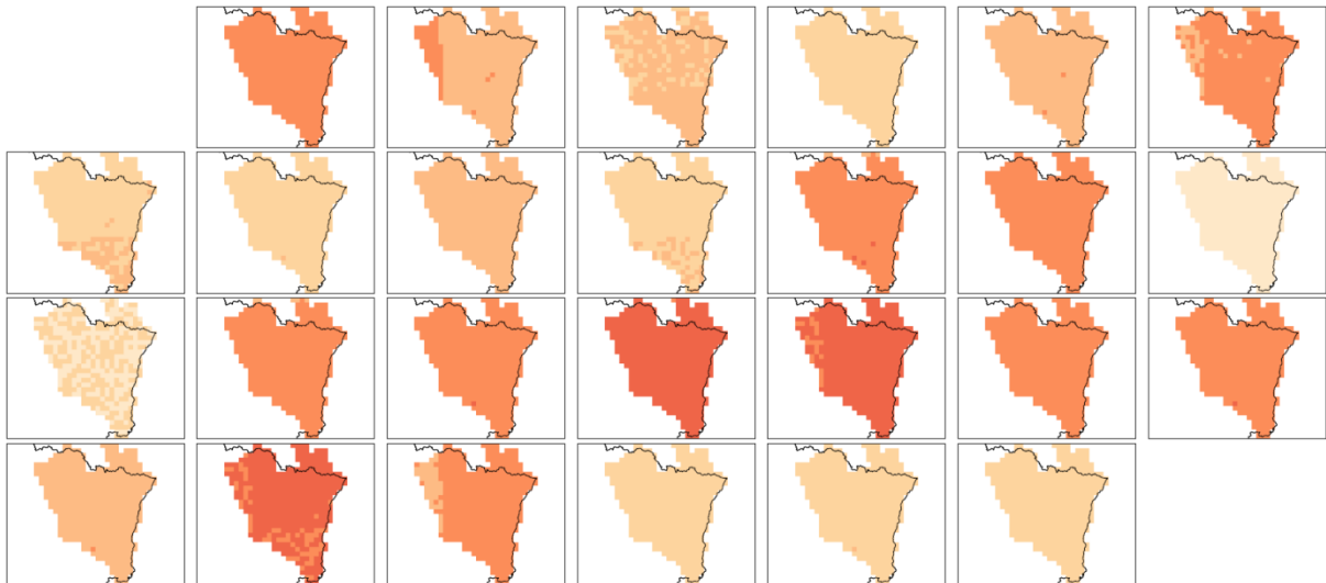
Figure 69 : Evolution de la température annuelle moyenne pour 26 modèles entre 2021-2050 et la période historique, données issues de l'ADC pour le RCP4.5.
