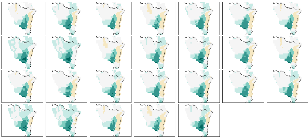
Figure 72 : Précipitation annuelle moyenne en mm/j pour 25 modèles, données issues de l'ADC pour le RCP8.5 pour la période 2021-2050. En haut à gauche la référence SAFRAN.
