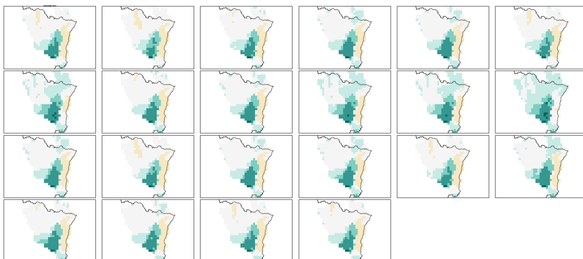
Figure 56 : Précipitation annuelle moyenne en mm/j pour 21 modèles, données issues de l'ADC pour le RCP2.6 pour la période 2021-2050. En haut à gauche la référence SAFRAN.
