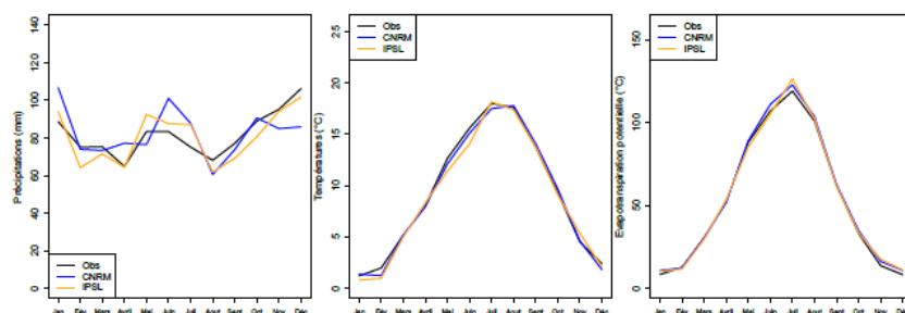
Figure 42 : Exemple de fiche climat pour la Moselle à Perl (partie supérieure, situation de référence).
