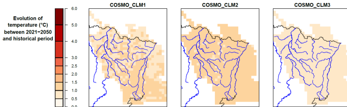
Figure 18 : Ecart de la température annuelle moyenne (°C) pour les trois réalisations du modèle COSMO-CLM entre 2021-2050 et la période de référence (1971-2000).
