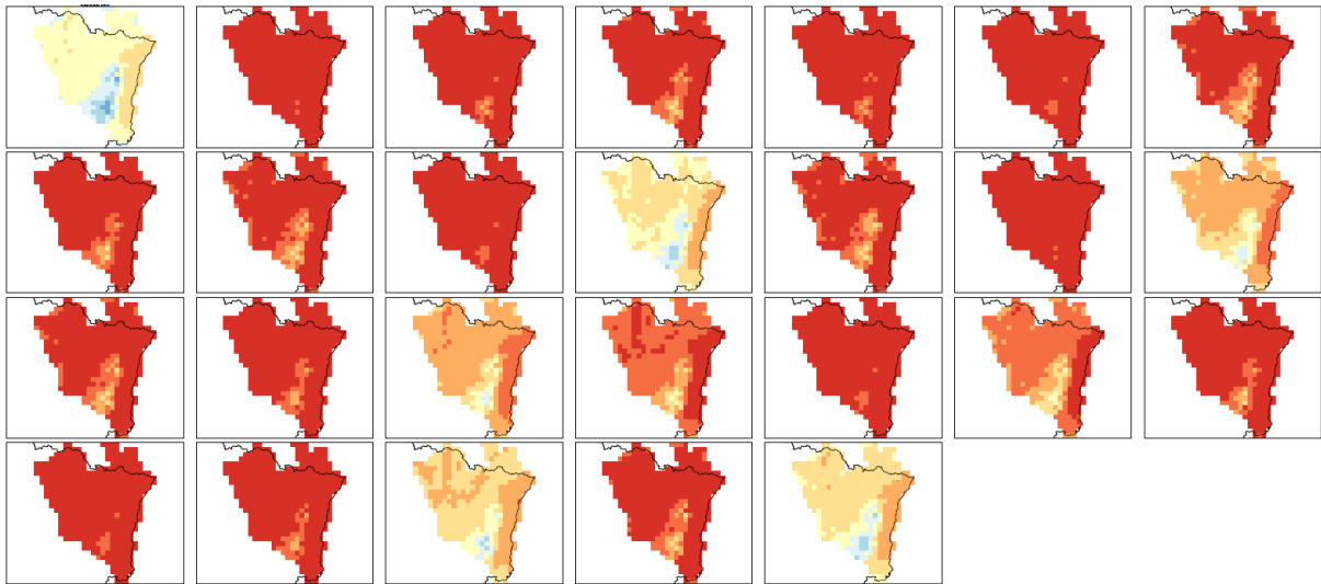
Figure 78 : Température annuelle moyenne pour 25 modèles, données issues de l'ADC pour le RCP8.5 pour la période 2071-2100. En haut à gauche la référence SAFRAN.
