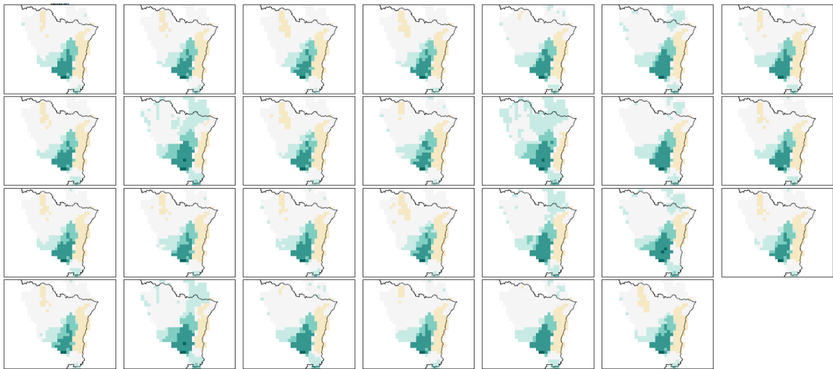
Figure 64 : Précipitation annuelle moyenne en mm/j pour 26 modèles, données issues de l'ADC pour le RCP4.5 pour la période 2021-2050. En haut à gauche la référence SAFRAN.
