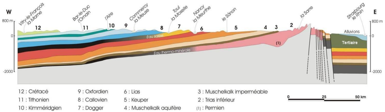
Illustration 8 - Coupe hydrogéologique schématique dans le bassin Rhin-Meuse (d'après Ramon et al., AERM, 1992)
