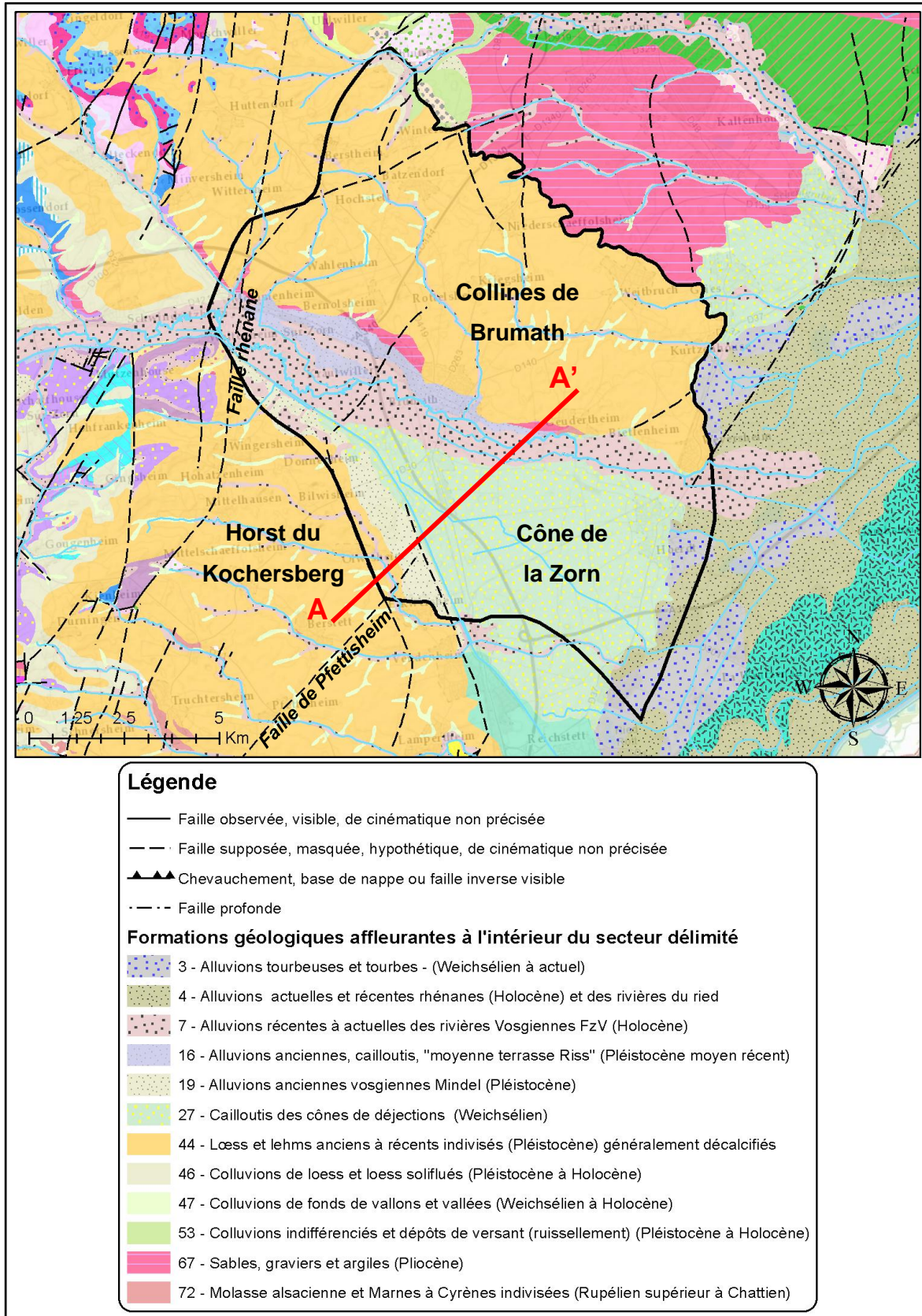
Illustration 32 : Extrait de la carte géologique au 1/50000 ème centrée sur le secteur « Mommenheim-Brumath-Cône de la Zorn » d'après la carte géologique de Brumath-DRusenheim (BRGM, 1972)
