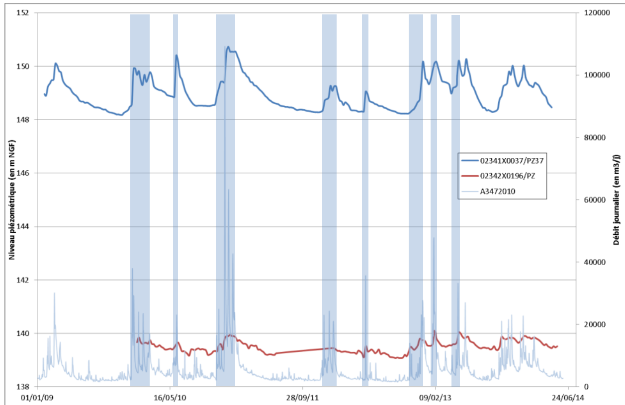
Illustration 50 : Chroniques piézométriques remarquables entre Mommenheim et Geudertheim et comparaison avec les débits enregistrés sur la Zorn dans la station hydrométrique de Waltenheim-sur-Zorn
