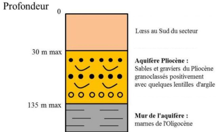
Illustration 37 : Coupes schématiques simplifiées des formations aquifères rencontrées au niveau des collines de Brumath (d'après APRONA, 2013)
