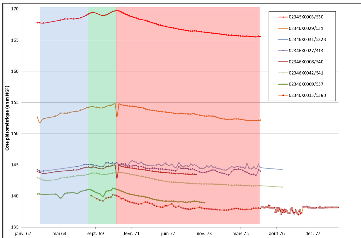
Illustration 23 : Comparaison des chroniques piézométriques de la partie amont du graben jusqu'à Lampertheim
