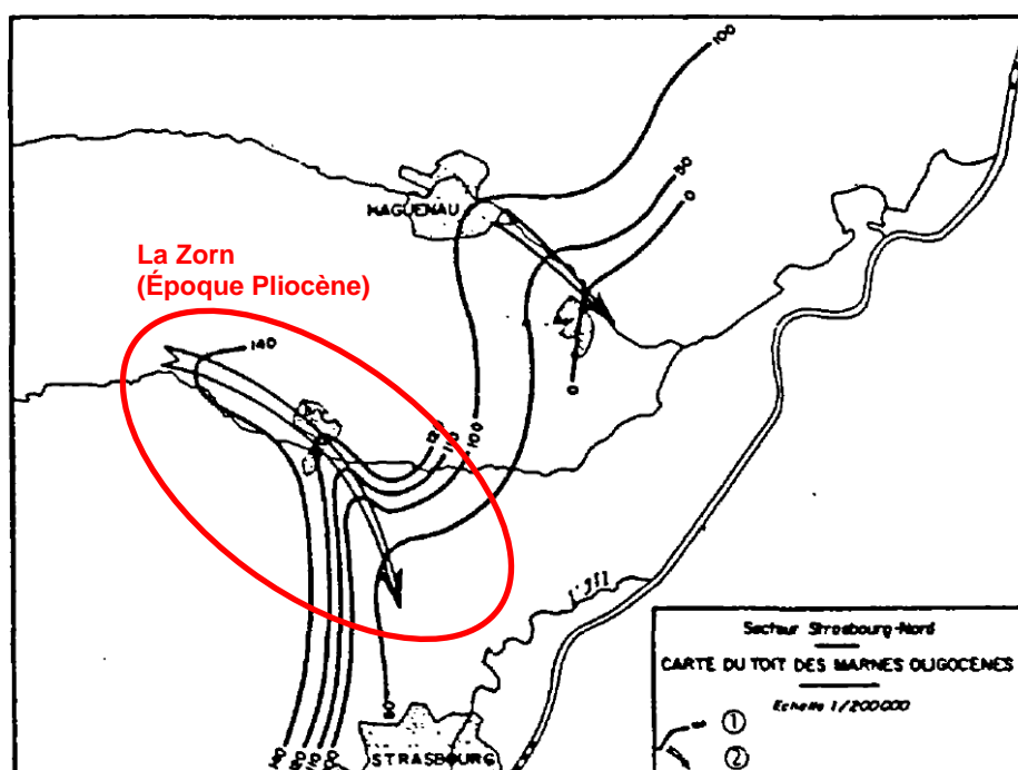
Illustration 33 : Paléovallées pliocènes dans la région de Strasbourg. Les courbes de niveau sont établies au toit de l'Oligocène. 1 : courbe de niveau du toit des marnes et sa cote, 2 : dépression (Simler et Millot, 1967)
