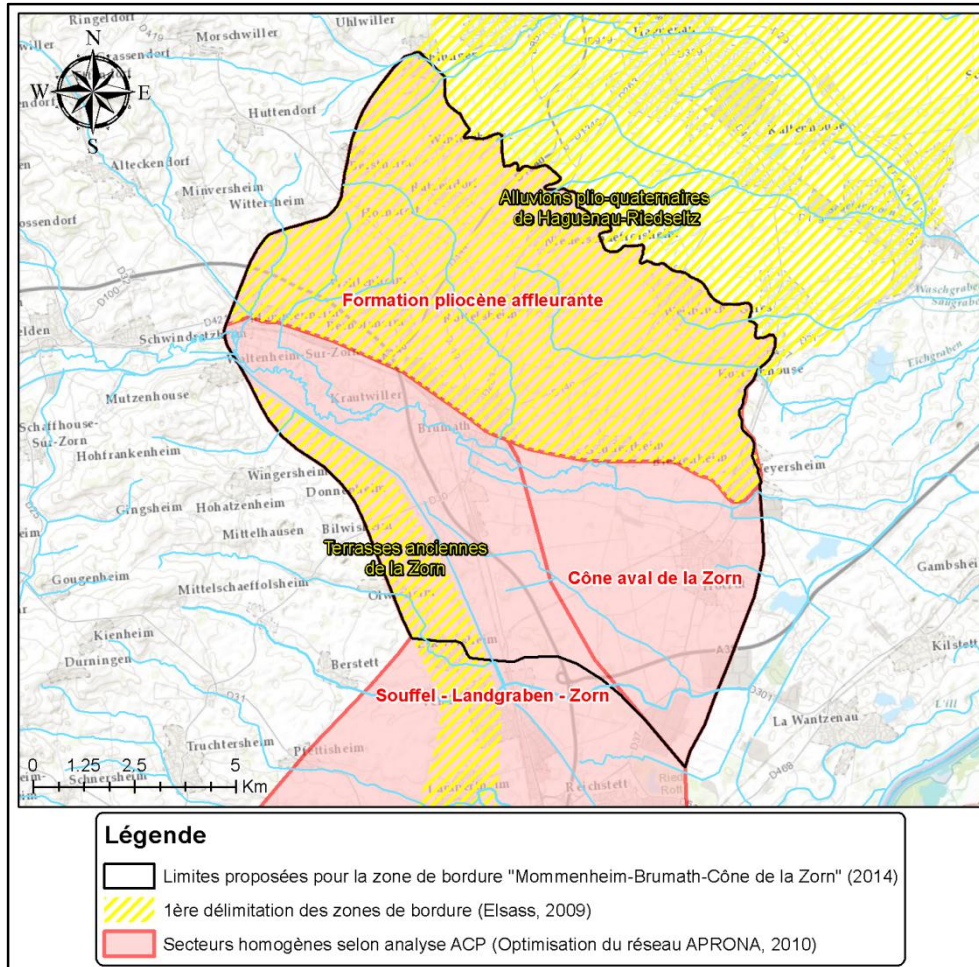
Illustration 30 : Les évolutions dans la définition d'un zonage homogène dans le secteur de la Zorn à travers trois études (Elsass, 2009 – Urban et al. , 2010 – Présente étude, 2014)
