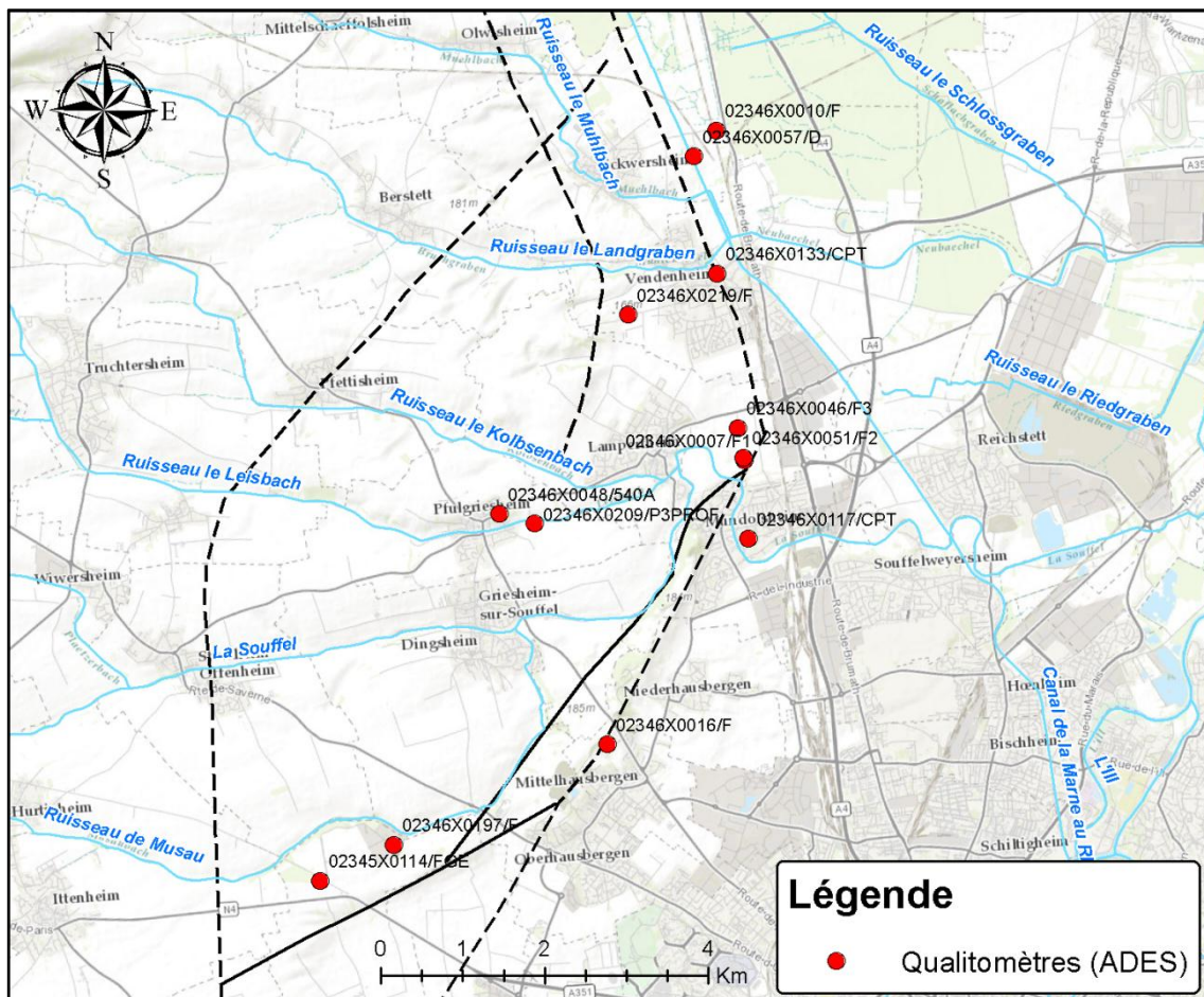
Illustration 24 : Localisation des qualitomètres ADES – graben de Pfulgriesheim
