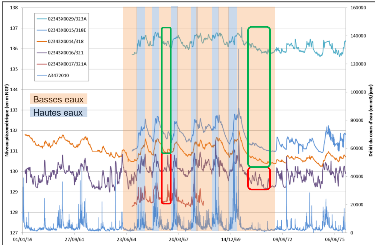
Illustration 51 : Chroniques piézométriques remarquables entre Mommenheim et Hœrdt et comparaison avec les débits enregistrés sur la Zorn dans la station hydrométrique de Waltenheim-sur-Zorn
