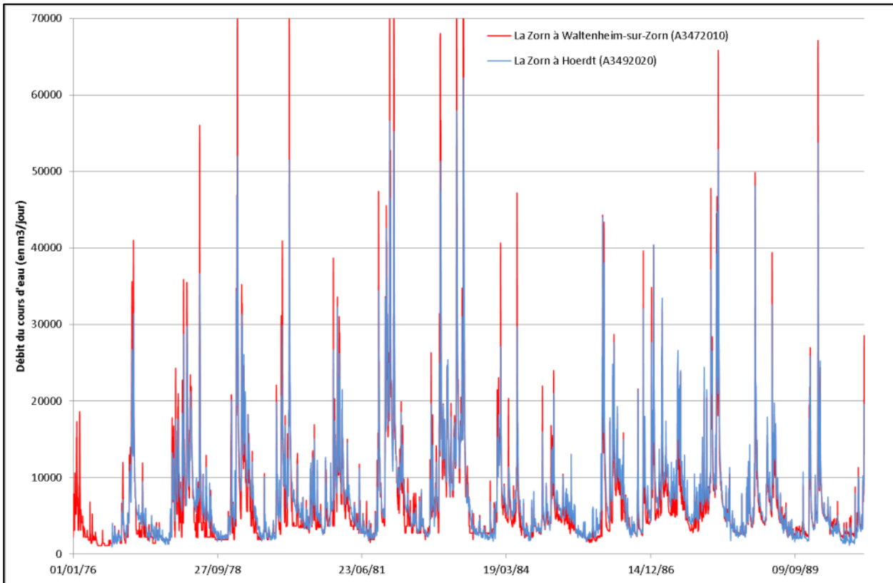
Illustration 42 : Comparaison des débits journaliers de la Zorn mesurés au niveau des stations de Waltenheim-sur-Zorn (amont) et d'Hœrdt (aval)
