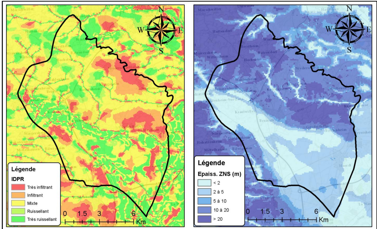
Illustration 55 : Comparaison IDPR et épaisseur de Zone Non Saturée – zone de « Mommenheim-Brumath-Cône de la Zorn »
