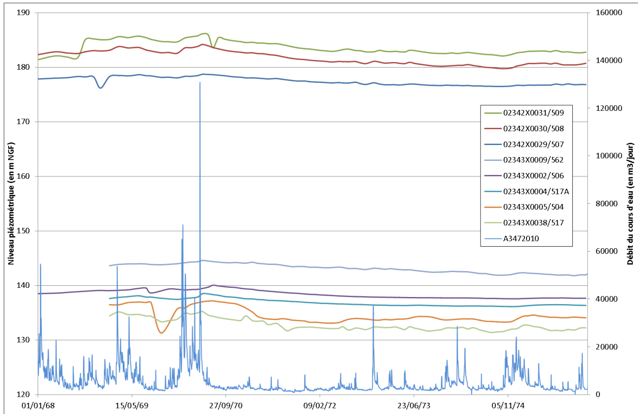
Illustration 48 : Chroniques piézométriques remarquables et comparaison avec les débits enregistrés sur la Zorn en amont – collines de Brumath (période 1968 à 1976)
