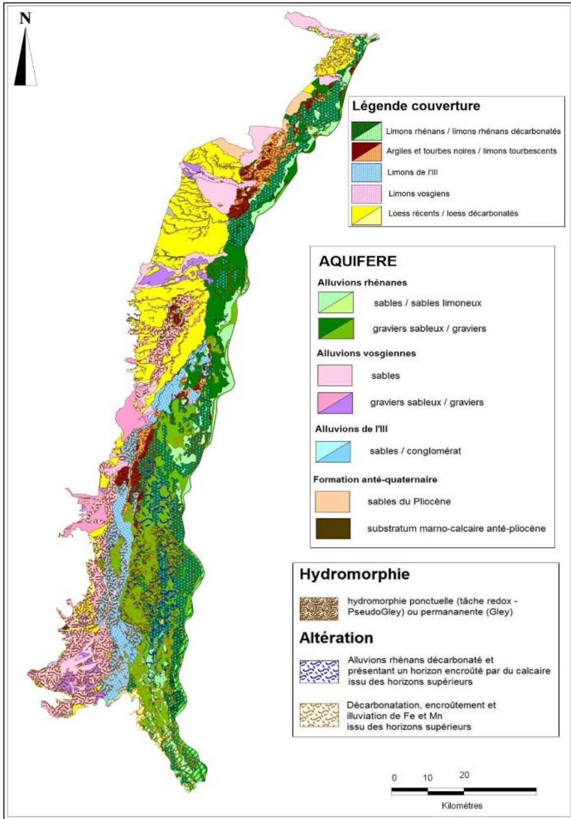
Illustration 1 : Cartographie des formations superficielles de la plaine d'Alsace (Urban et Boucher, 2011 - Programme BRAR Région Alsace 2011-2014)
