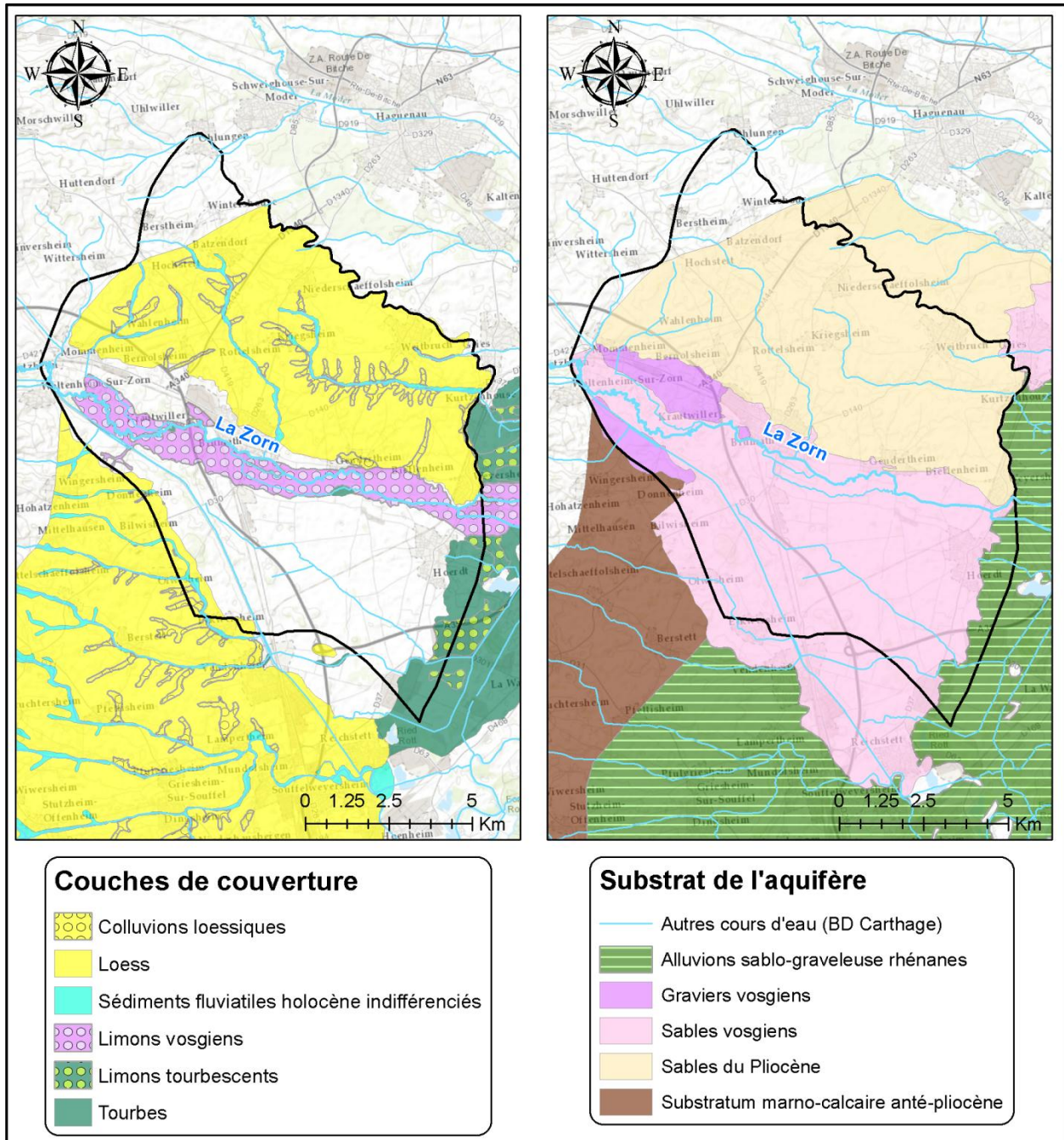
Illustration 35 : Cartographie des formations superficielles dans la zone Mommenheim-Brumath-Cône de la Zorn - à gauche, les formations récentes de couverture, à droite le substrat des formations aquifères (d'après Urban et Boucher, 2011)
