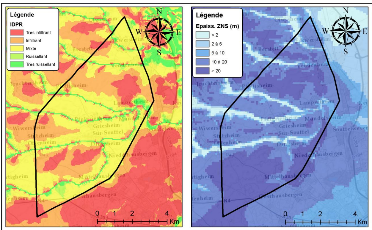
Illustration 27 : Comparaison IDPR et épaisseur de Zone Non Saturée – zone du « graben de Pfulgriesheim »
