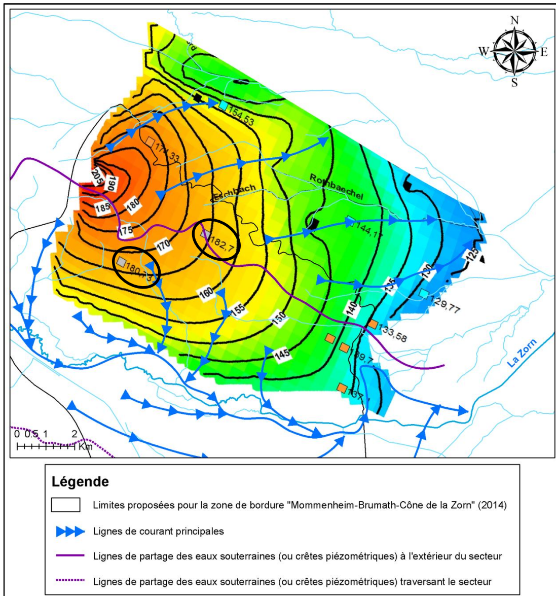
Illustration 40 : Comparaison des lignes de courants principales calculées à partir de la grille d'épaisseur moyenne de la zone non saturée avec la carte piézométrique simulée issue du modèle hydrodynamique de la nappe du Plio-Quaternaire (APRONA, 2013)
