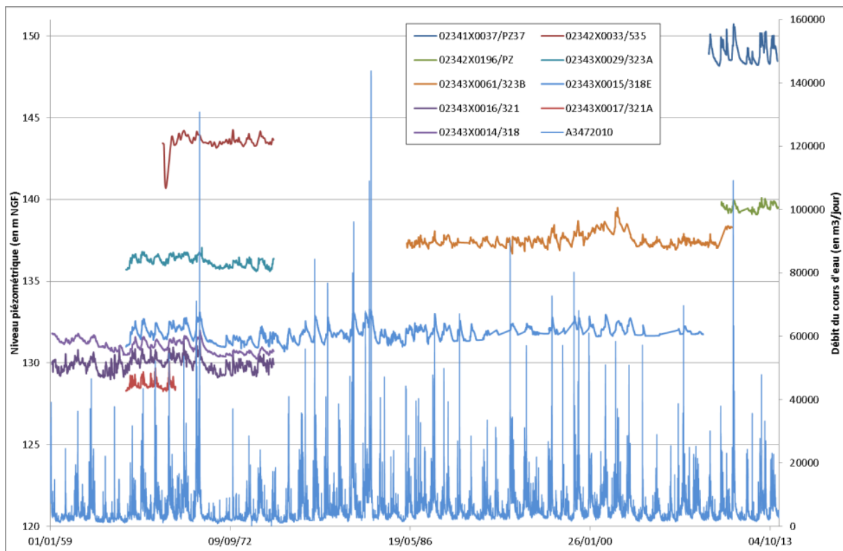
Illustration 49 : Chroniques piézométriques remarquables d'ouvrages le long de la Zorn et comparaison avec les débits enregistrés sur la Zorn en amont
