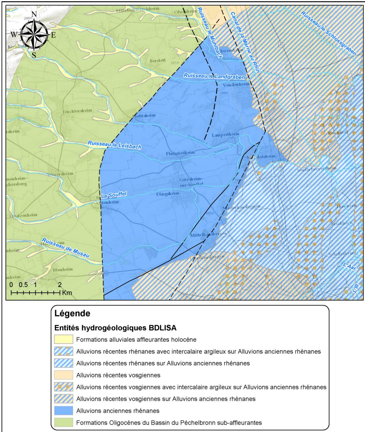
Illustration 15 : Cartographie des entités hydrogéologiques affleurantes du référentiel BDLISA répertoriés dans le graben de Pfulgiesheim
