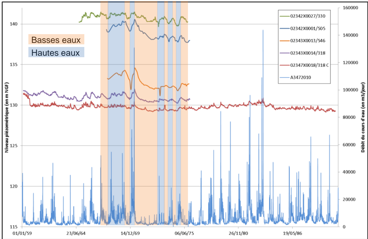
Illustration 52 : Chroniques piézométriques remarquables au sein du cône de déjection et comparaison avec les débits enregistrés sur la Zorn dans la station hydrométrique de Waltenheim-sur-Zorn
