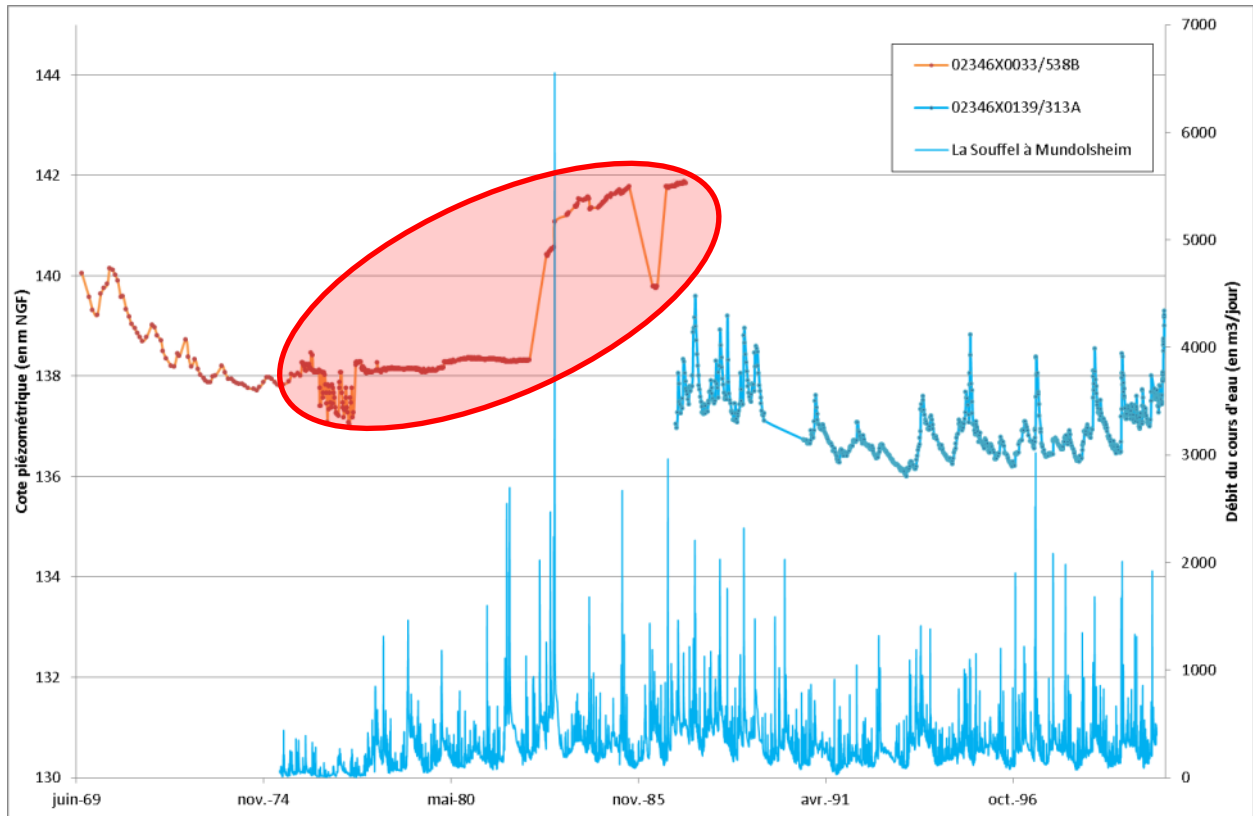
Illustration 22 : Comparaison des chroniques piézométriques des deux points d'eau à chronique longue situés à Lampertheim avec la chronique de débits journaliers enregistrés par la station hydrométrique de la Souffel à Mundolsheim
