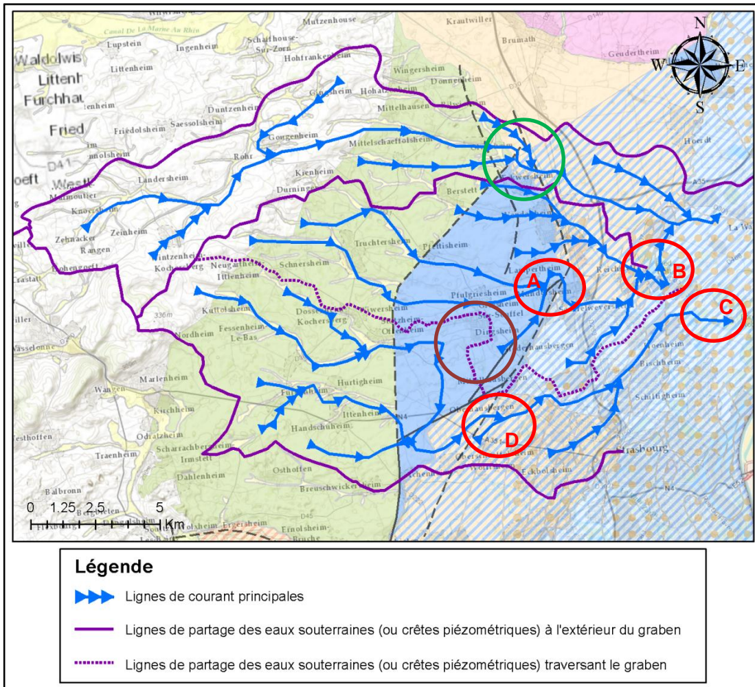
Illustration 16 : Localisation des lignes de courant principales et des lignes de partage des eaux souterraines – graben de Pfulgriesheim
