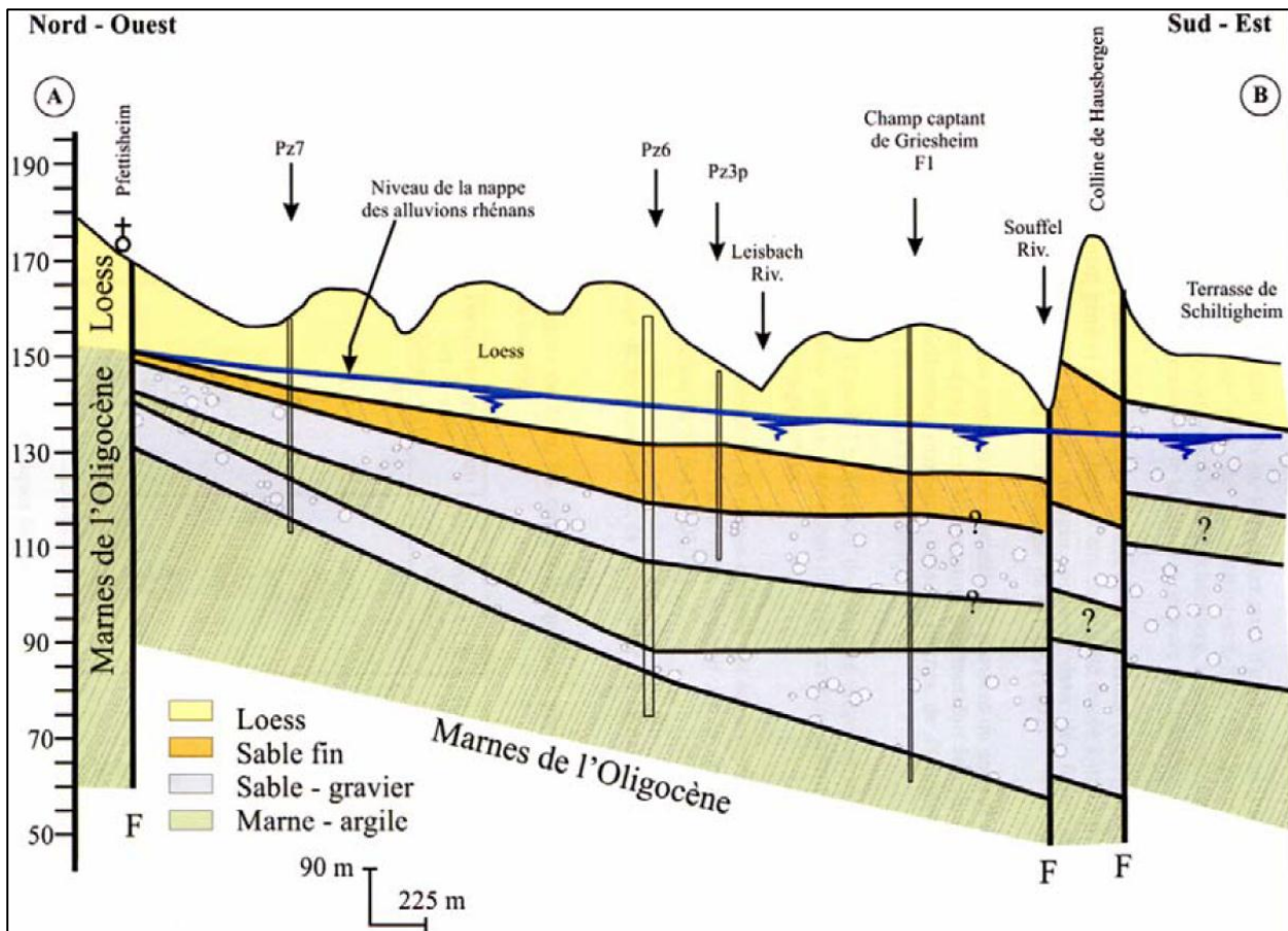
Illustration 13 : Coupe schématique Nord-Ouest/Sud-Est du graben de Pfulgriesheim (Frey, 2006)
