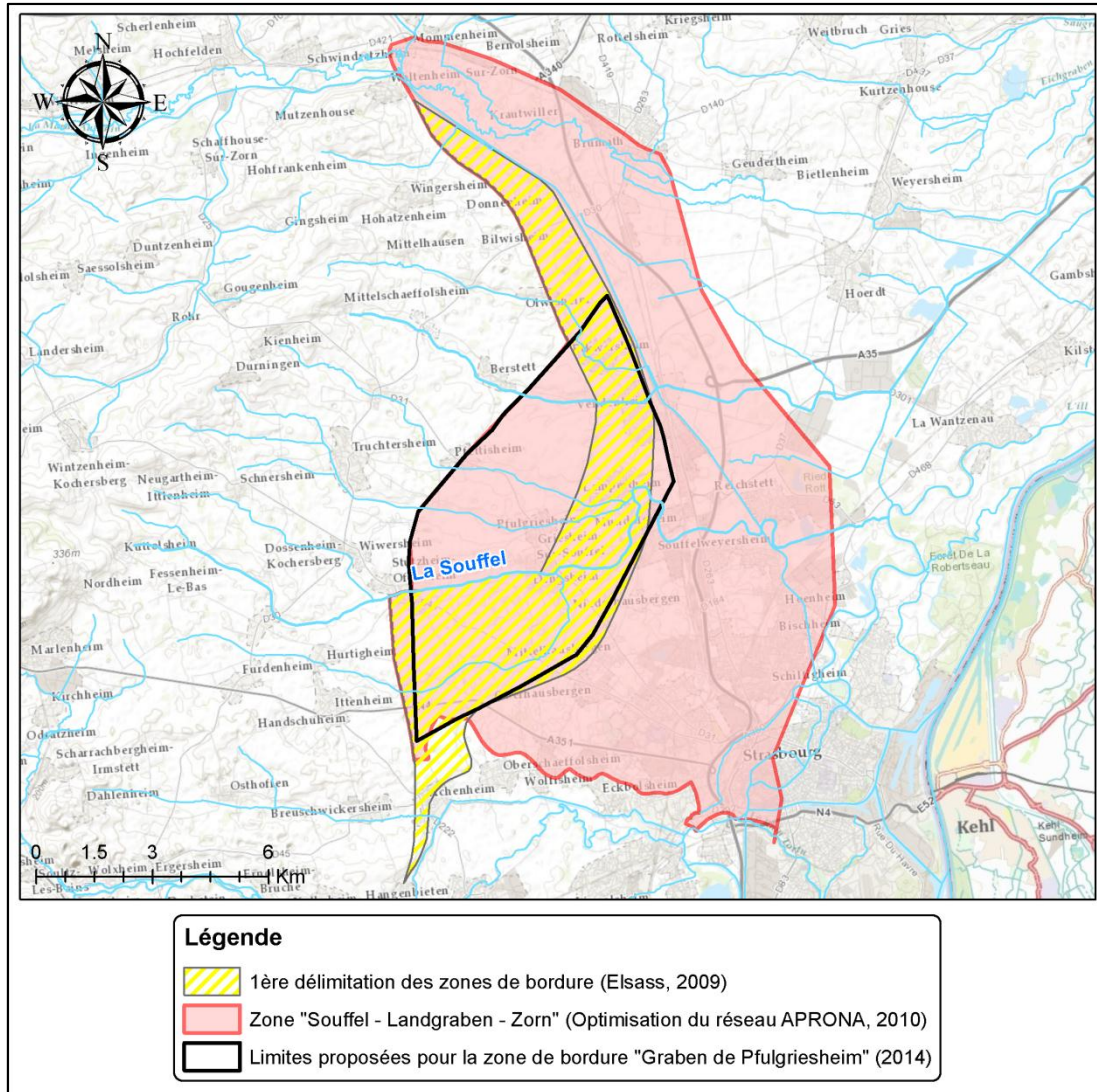
Illustration 11 : Les évolutions dans la définition d'un zonage homogène dans le secteur du graben de Pfulgriesheim à travers trois études (Elsass, 2009 – Urban et al. , 2010 – Présente étude, 2014)
