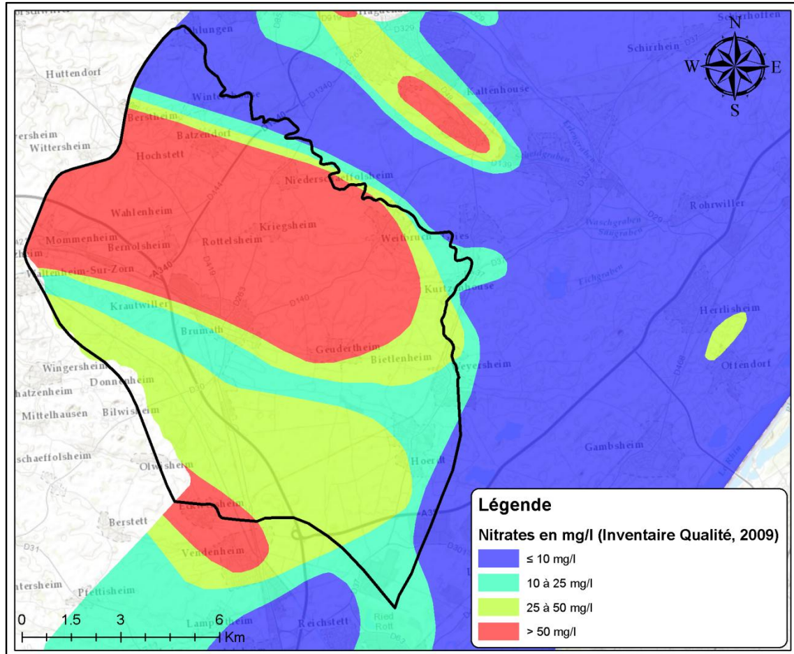
Illustration 56 : Carte des concentrations en nitrates dans les eaux souterraine issue de l'Inventaire de la qualité des eaux souterraines dans le Fossé Rhénan – zone de « Mommenheim-Brumath-Cône de la Zorn » (Région Alsace, 2012)
