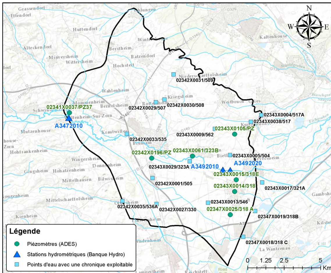
Illustration 47 : Localisation des piézomètres ADES et hors ADES et des stations de mesure hydrométrique référencées dans la Banque Hydro – secteur « Mommenheim-Brumath-Cône de la Zorn »
