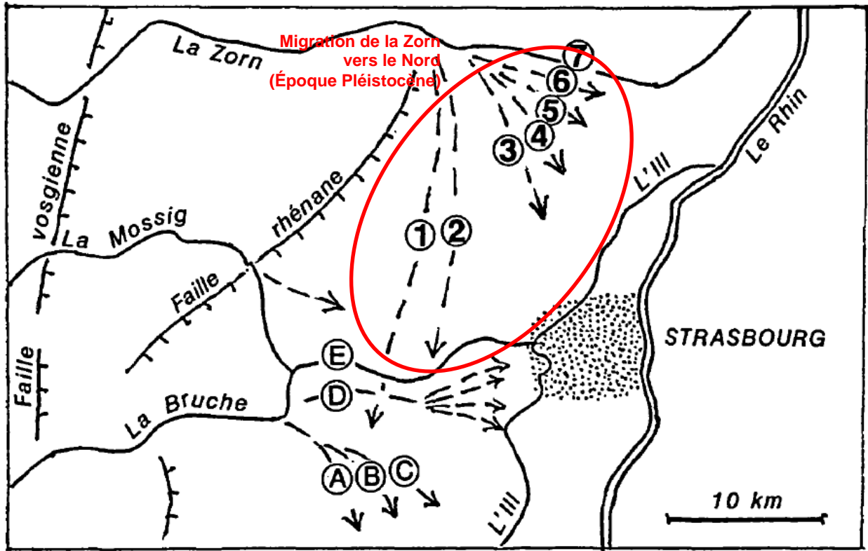
Illustration 34 : Migration du cours de la Zorn (1 à 7) vers le Nord, au cours du Quaternaire (d'après Vogt, 1992)
