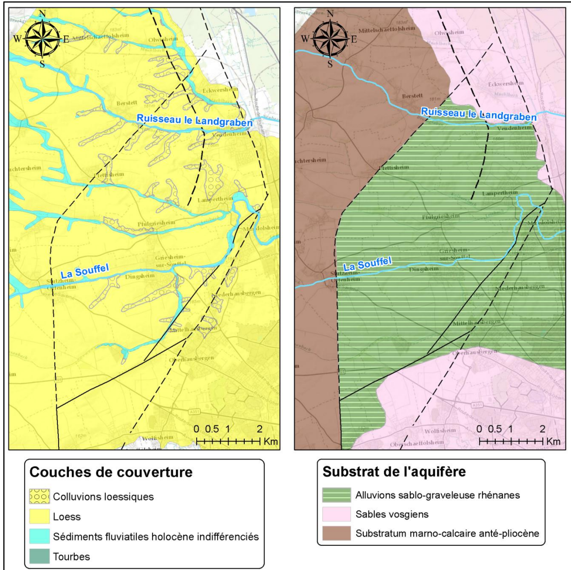
Illustration 14 : Cartographie des formations superficielles dans la zone du graben de Pfulgriesheim - à gauche, les formations récentes de couverture, à droite le substrat des formations aquifères (d'après Urban et Boucher, 2011)
