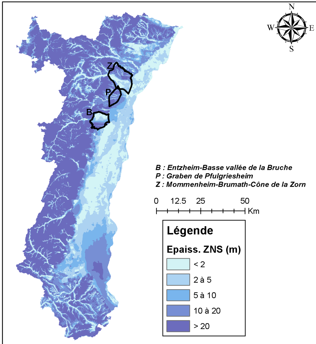
Illustration 2 : Grille d'épaisseur de ZNS en région Alsace (d'après Allier et al., 2011)
