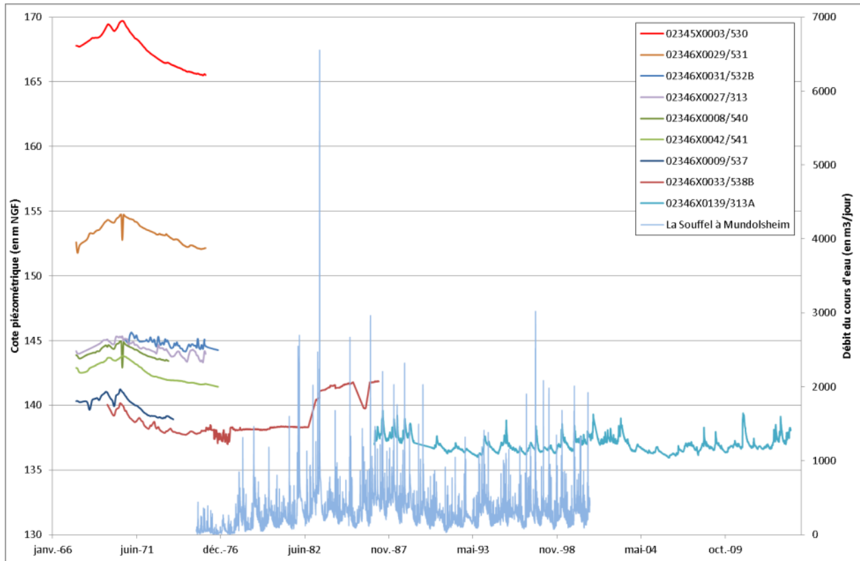
Illustration 21 : Chroniques piézométriques remarquables et comparaison avec les débits enregistrés sur la station hydrométrique la plus proche – graben de Pfulgiesheim
