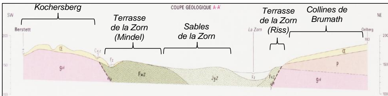
Illustration 31 : Coupe géologique traversant le cône de déjection de la Zorn, entre les villages de Berstett et de Geudertheim (carte géologique au 1/50000 ème , BRGM, 1972)
