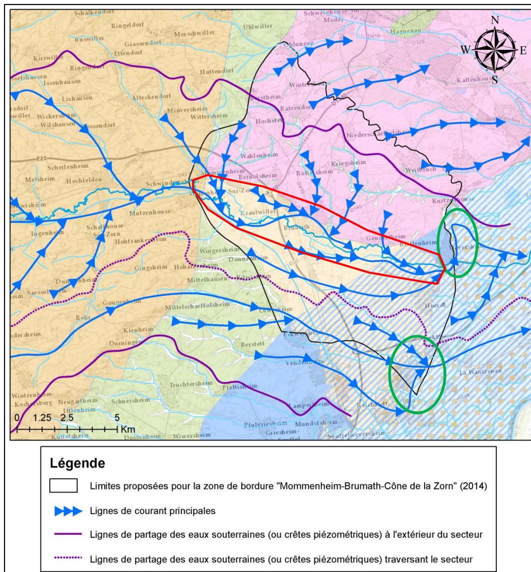
Illustration 39 : Localisation des lignes de courant principales et des lignes de partage des eaux souterraines – Mommenheim-Brumath-Cône de la Zorn
