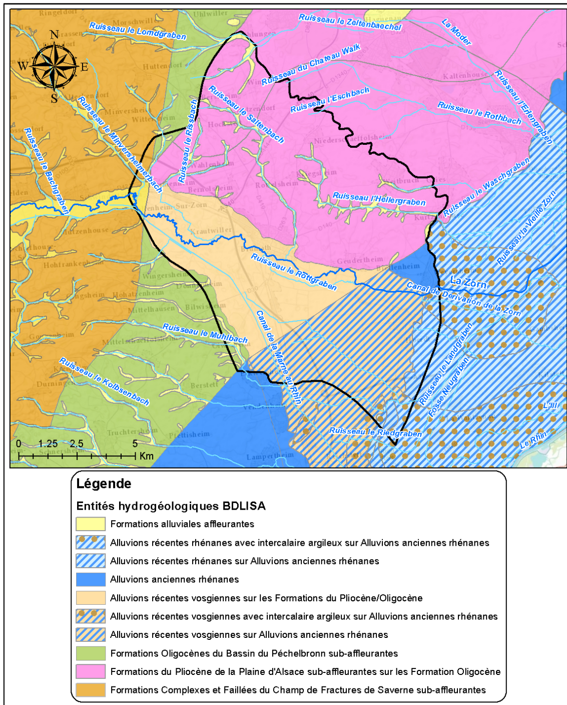
Illustration 36 : Cartographie des entités hydrogéologiques affleurantes du référentiel BDLISA répertoriés dans le secteur d'étude « Mommenheim-Brumath-Cône de la Zorn »
