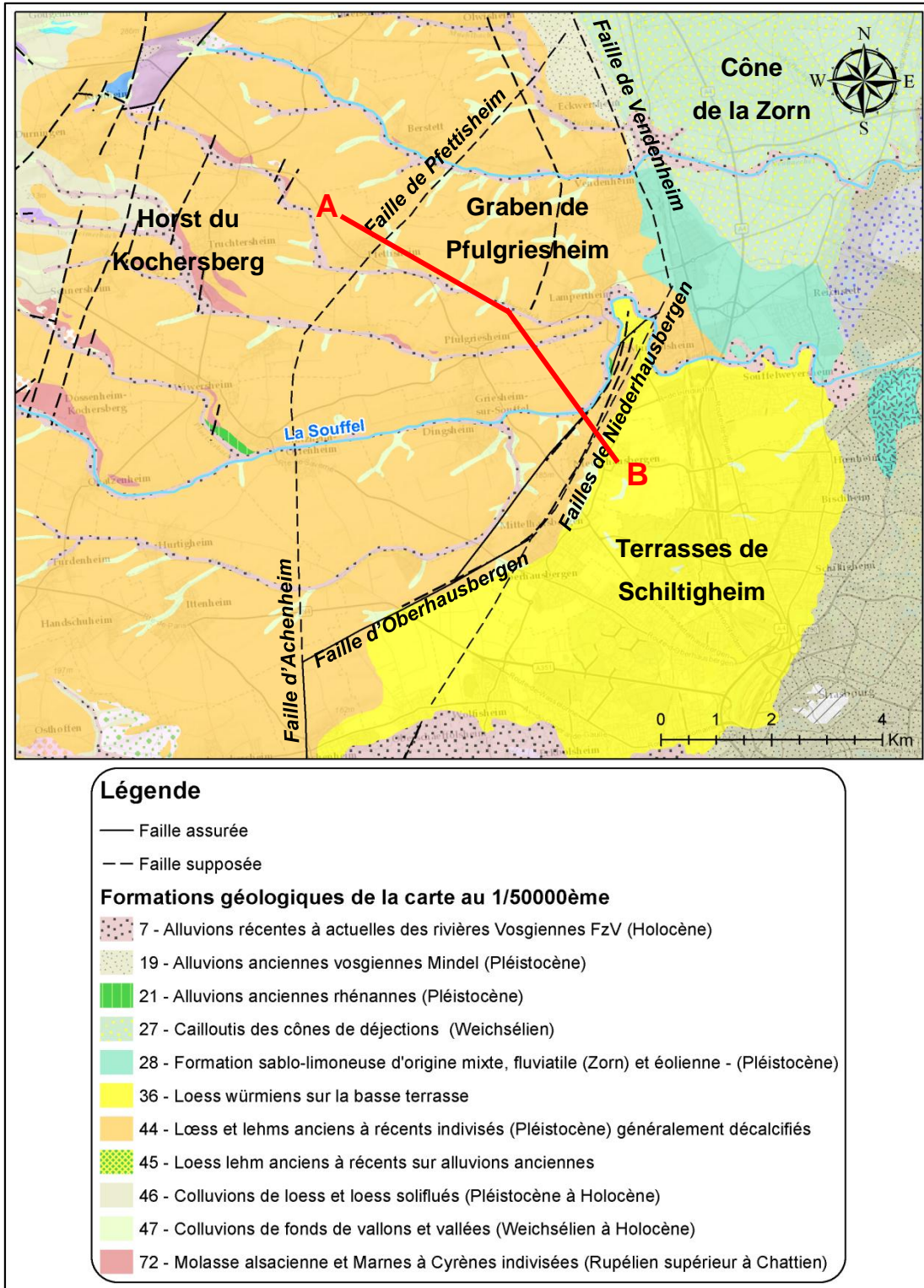
Illustration 12 : Carte géologique au 1/50000 ème centrée sur le graben de Pfulgriesheim (trait rouge = coupe schématique réalisée par Frey en 2006)
