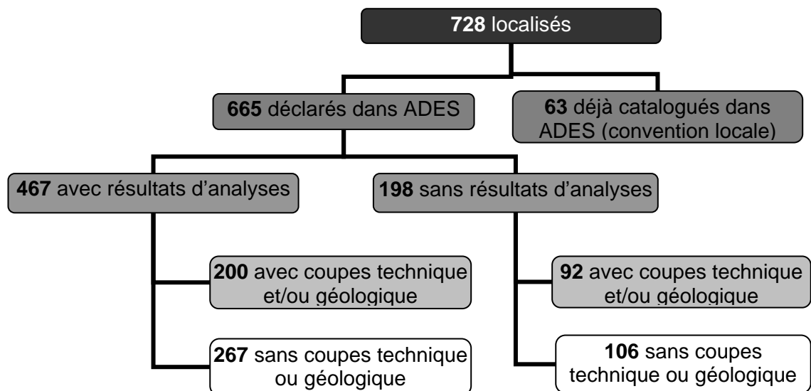
Illustration 3 : Logigramme présentant les 728 forages recensés dans les dossiers des ICSP
