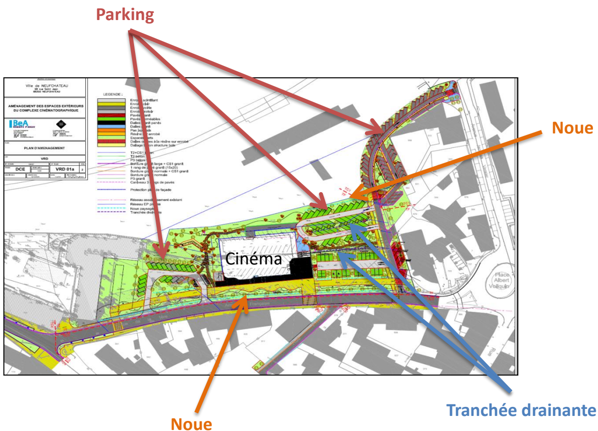
Zone d'infiltration des eaux pluviales
